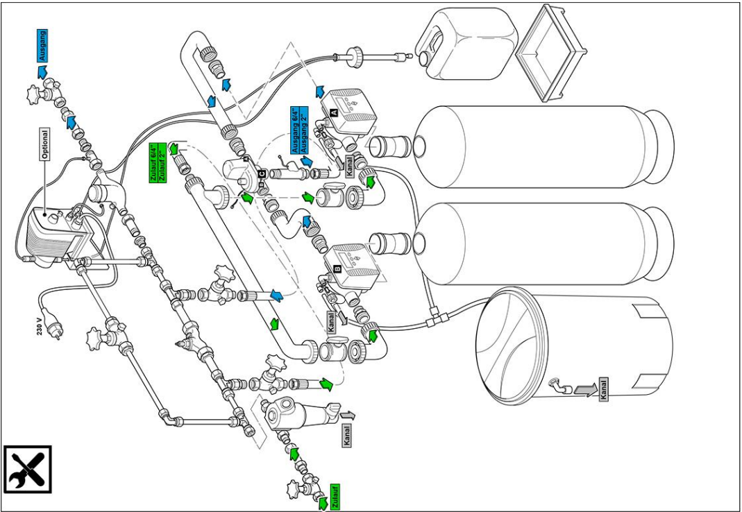
Pendel-Enthärtung_EHPD_040-0400bis1000_050-0600bis1000_Verschneidventil.iso
